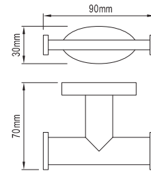
Double Robe Hook 113169
